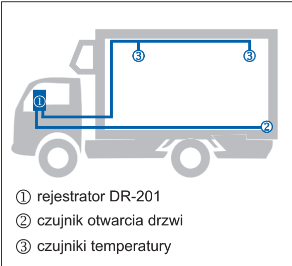
Rys.1 Przykład instalacji rejestrującej w samochodzie ciężarowym.
