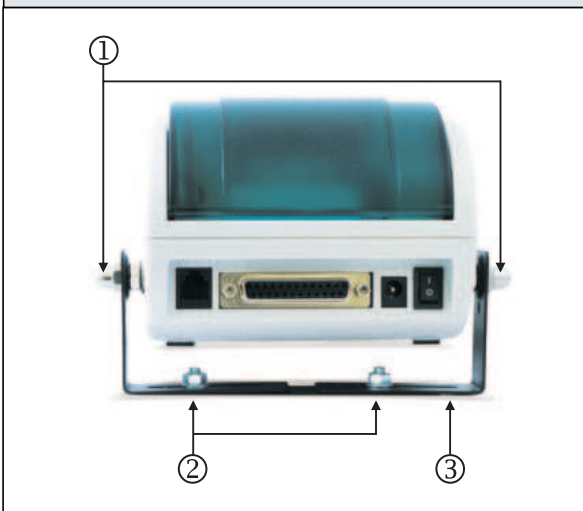
Rys.2 Uchwyt montażowy (3).
